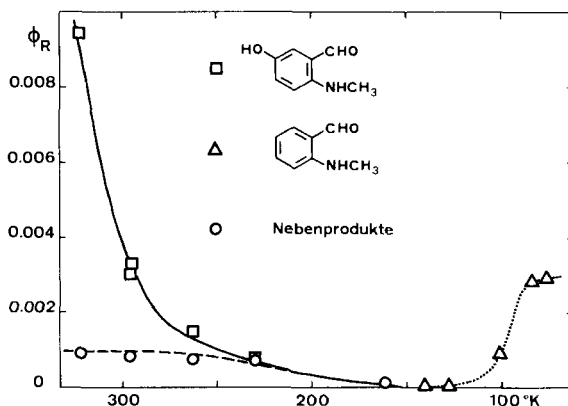
Fig. 3. Temperaturabhängigkeit der Quantenausbeuten photochemischer Umwandlungen von 2-Äthyl-1-methyl-indazolium-tetrafluoroborat (EMI) in 95% Äthanol
