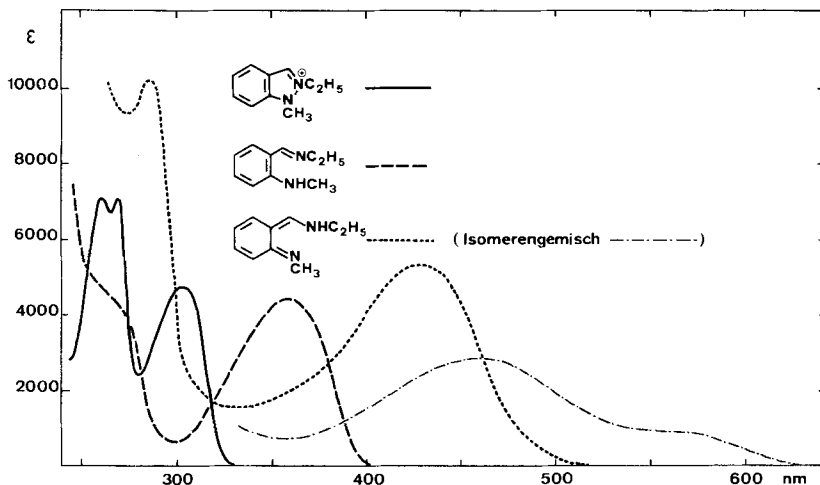
Fig. 2. Tieftemperatur-Photochemie von 2-Äthyl-1-methyl-indazolium-tetrafluoroborat (EMI) ————— UV.-Spektrum von EMI in Äthanol
