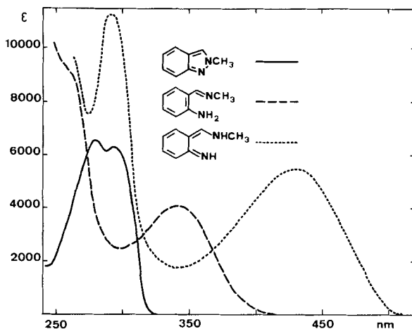
Fig. 1. Tieftemperatur-Photochemie von 2-Methyl-indazol ( 1a )
